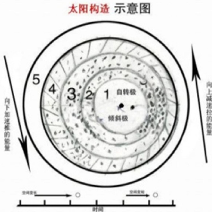
此图是太阳轴极构造,各点表示微粒和离子分布,切线表示光球若干活动线 1、日核以 1500 万度向 2 中介层向 3 对流层向 4 光球 6000 度外辐射对流,五 色球也是以 1500 万度从外向内辐射对流从此改变离子质量。
