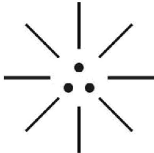
(Fundamental Neutrinos)
