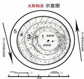
此图是太阳构造示意图, 各点表示米粒和原子分布, 切线表示光球层平流运动 1. 自转以 1500 万度向 2 中角向 3 对旋向 4 空球 6000 度外辐射对旋, 五 色球也是以 1500 万度从外向内辐射对旋从此改变原子质量。
