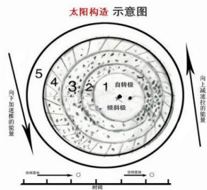
图2 太阳原始构造物理图像
