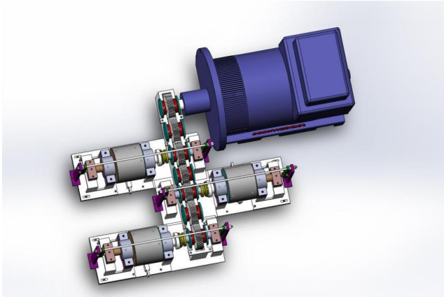
组合式偏心涡旋发动机
