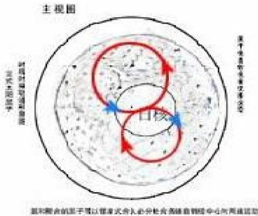
原子核由原子核以核力式向中心必社会核力核力中心向核力核力
