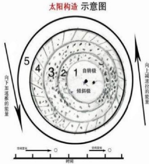
此图是太阳的构造,各点表示微粒和离子分布,切线表示光球若干活动线 1、日核以1500万度向2中介质向3对流层向4光球6000度外辐射对流,五色球也是以1500万度从外向内辐射对流从此改变原子质量。
