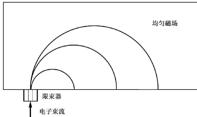
图 1. 不同能量电子在均匀磁场中运动轨迹的实验
