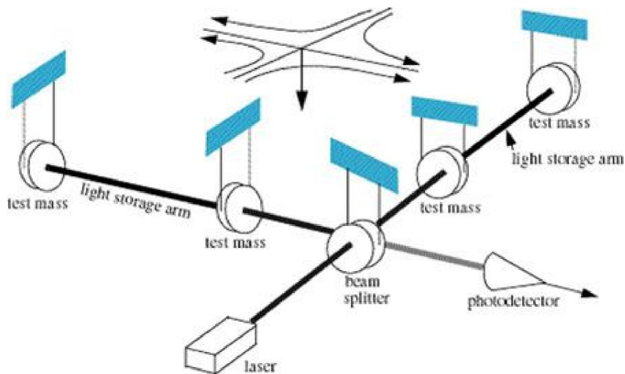
LIGO 探测器图示
