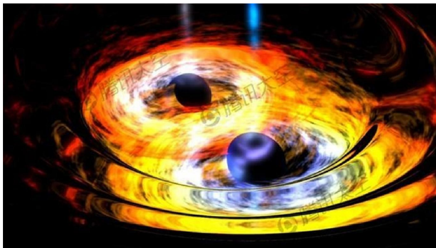
两颗黑洞相互盘旋发出引力波示意图
