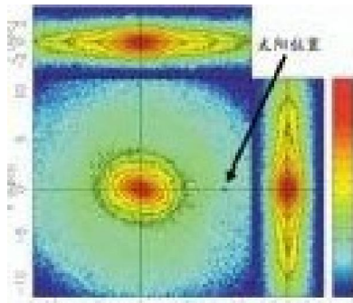
根据最新模型,银河系棒的长度应该是约 2.5 万光年左右,与太阳—银心方向成约 20 度角。
