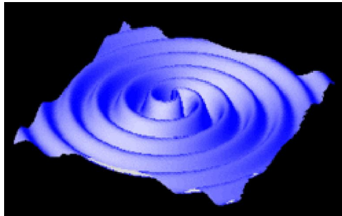
引力波——时空的波纹（示意图）
