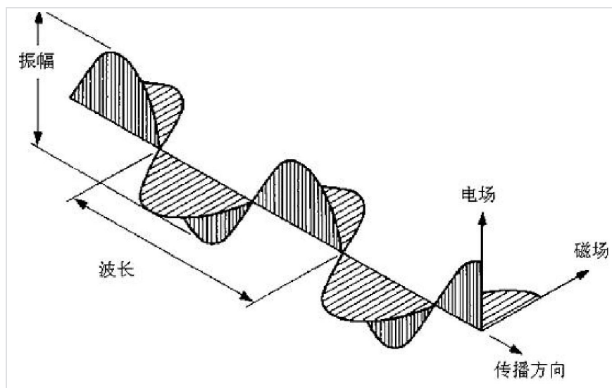
图 1. 麦克斯韦光波的电场和磁场
