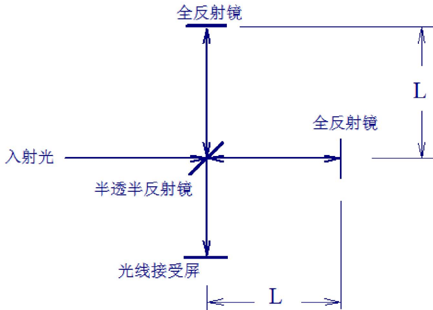
图 1. 迈克尔逊干涉光路示意图
