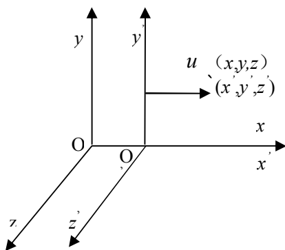
图1 洛伦兹变换
