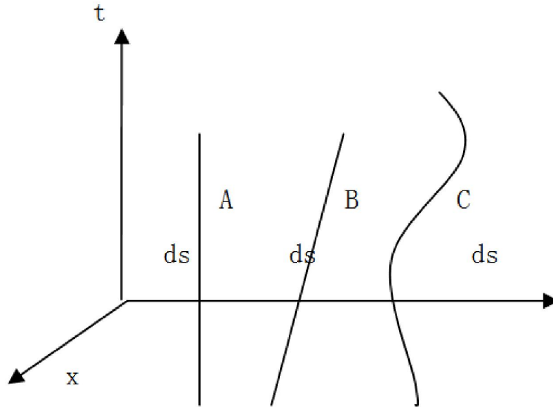
图 1 四维时空中的世界线 ds^2 = 0 \Leftrightarrow v^2 = c^2 类时间隔 时空中任取一点 p，与 p 的间隔类光的点组成如图 2 所示的锥面，成为 p 点的光锥。
