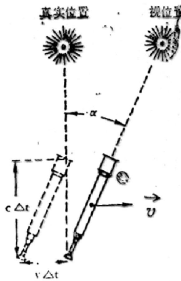
如图: [布喇德雷光行差现象](1728)
