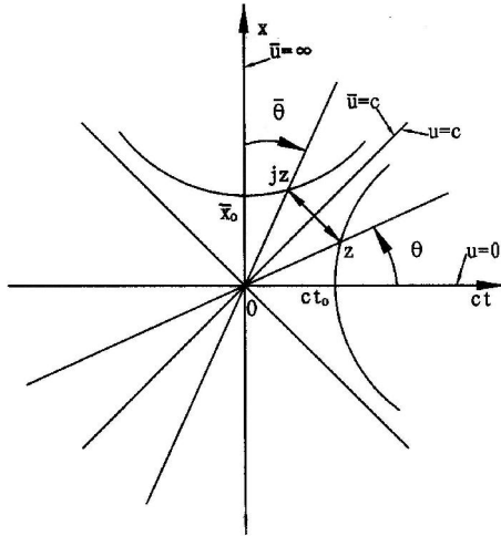
图 1. 新时空理论
