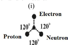
(ATOM)
