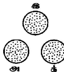
(Species Neutrinos)
